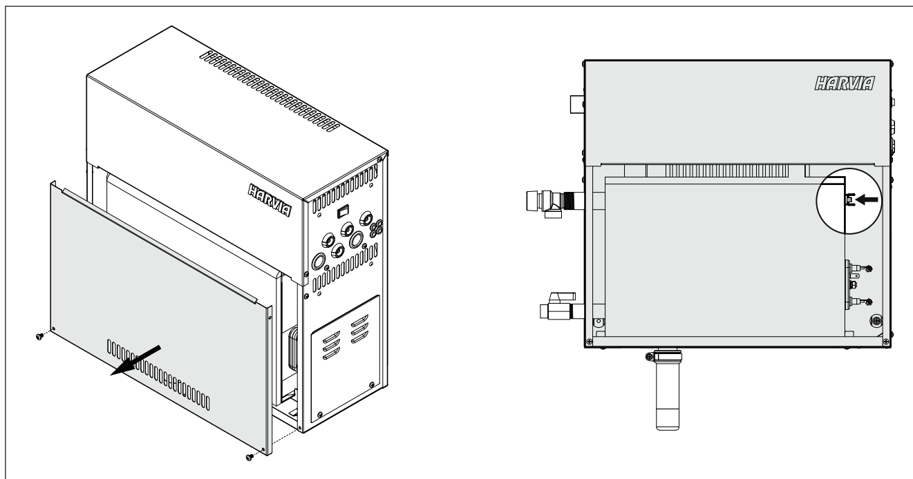
Figure 9. Réinitialiser le fusible de surchauffe Figuur 9. De beveiliging tegen oververhitting resetten
